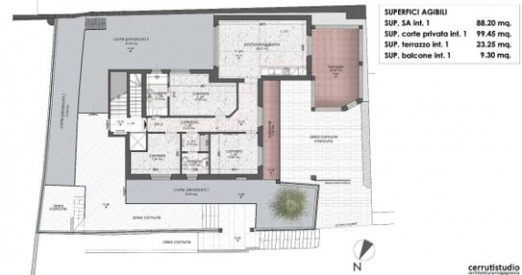
PLANIMETRIA - STATO DI PROGETTO PIANTA PIANO TERRA scala 1:100
